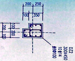
DZ2配筋图
