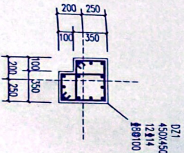
DZ1配筋图
