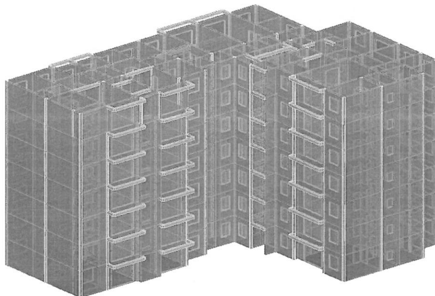
图 4-1 房屋结构计算模型
