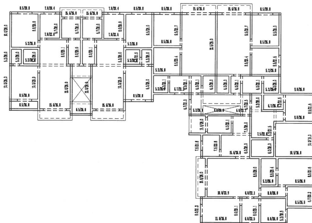
图 6.5-1 一层墙高厚比计算简图
