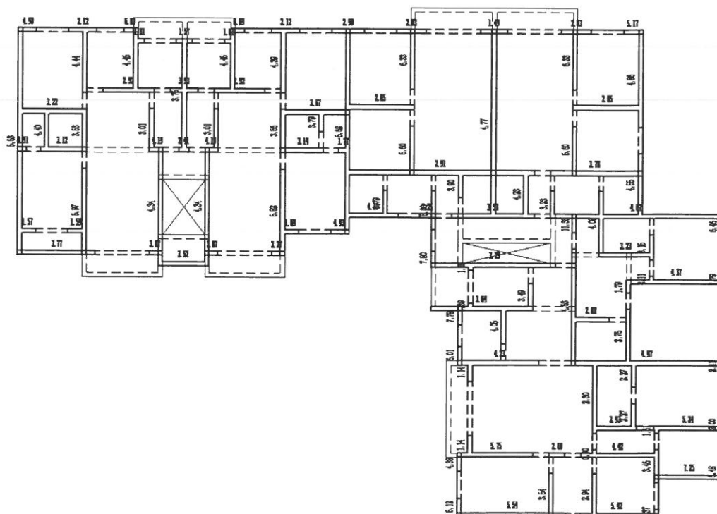
图 6.4-4 四层墙体受压承载力计算简图
