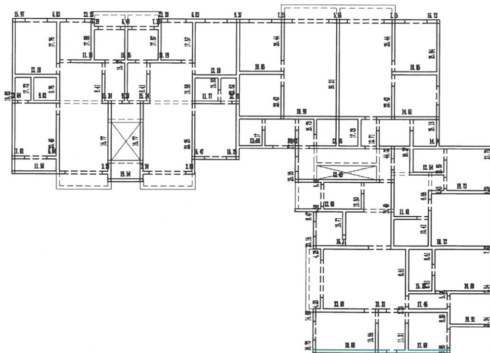
图 6.4-7 七层墙体受压承载力计算简图
