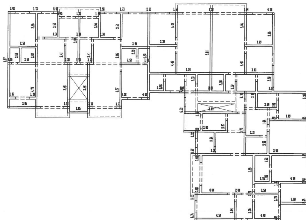
图 6.4-3 三层墙体受压承载力计算简图
