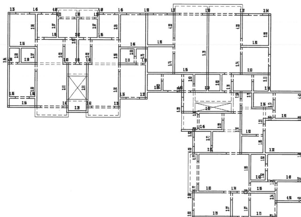
图 6.4-2 二层墙体受压承载力计算简图
