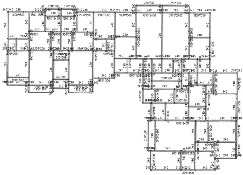
图 6.2-1 一层结构平面简图
