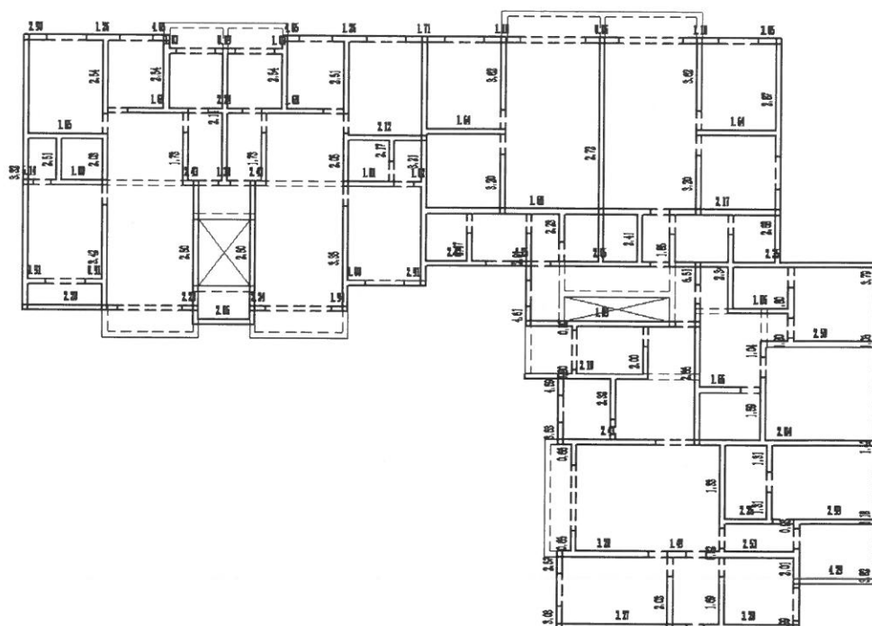
图 6.4-1 一层墙体受压承载力计算简图
