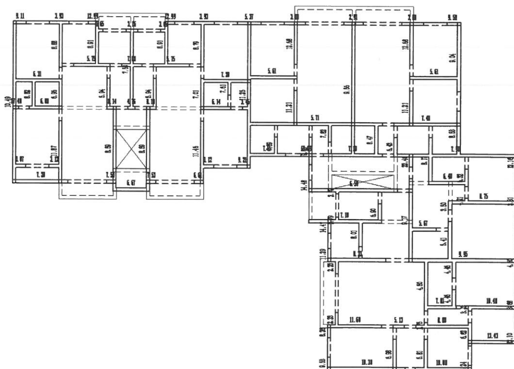
图 6.4-6 六层墙体受压承载力计算简图
