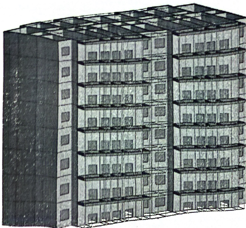
图 4-1 结构验算计算模型
