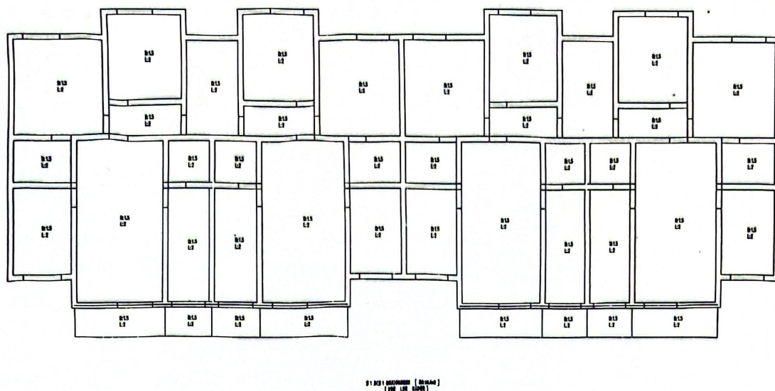
图 4-10 1 层楼板荷载简图
