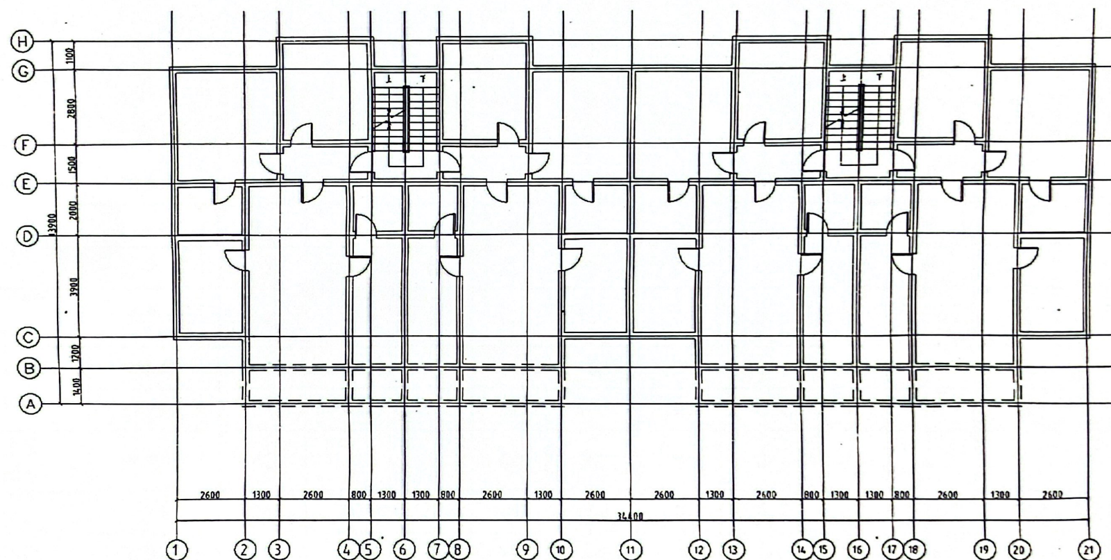
1-8 层平面布置图
