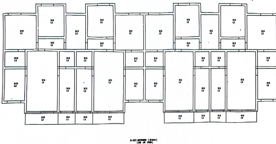
图 4-15 6 层楼板荷载简图
