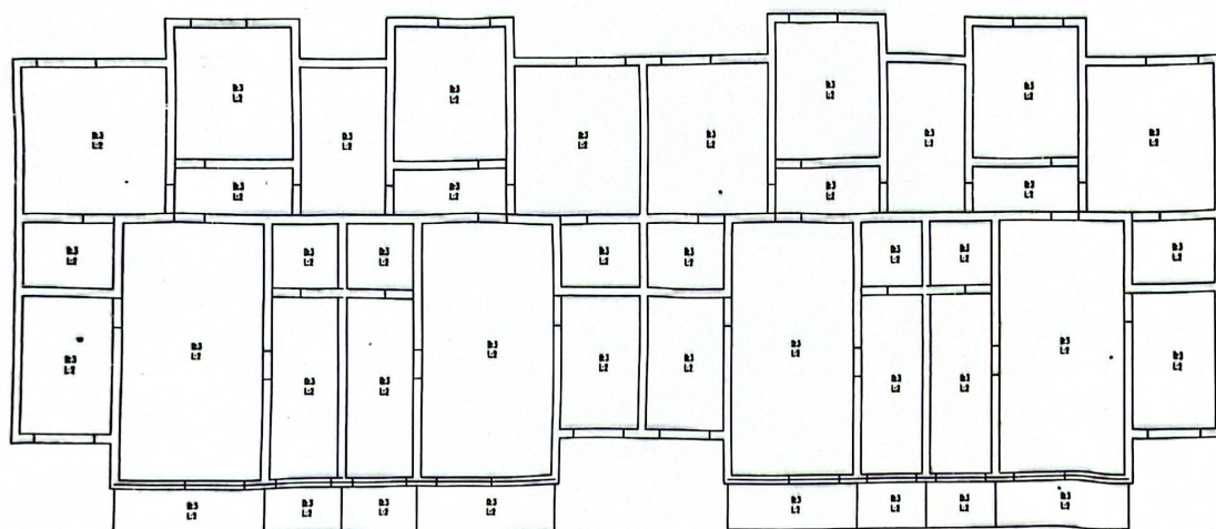
图 4-16 7 层楼板荷载简图
