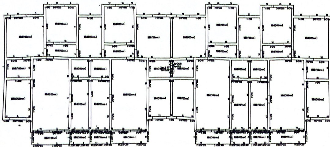
图 4-8 7 层结构平面简图
