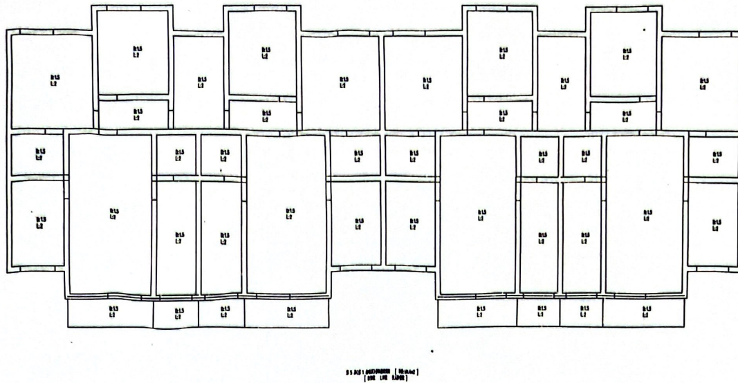
图 4-14 5 层楼板荷载简图
