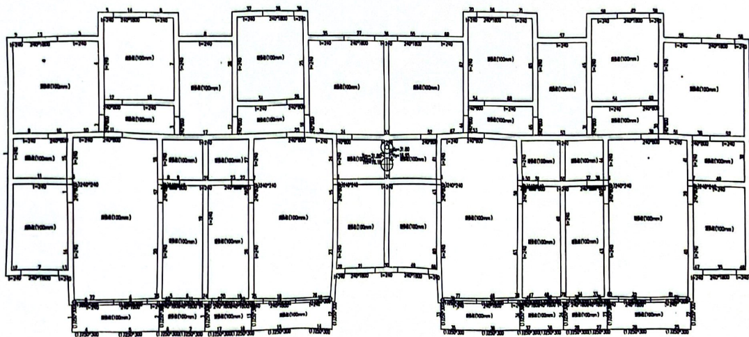
图 4-6 5 层结构平面简图
