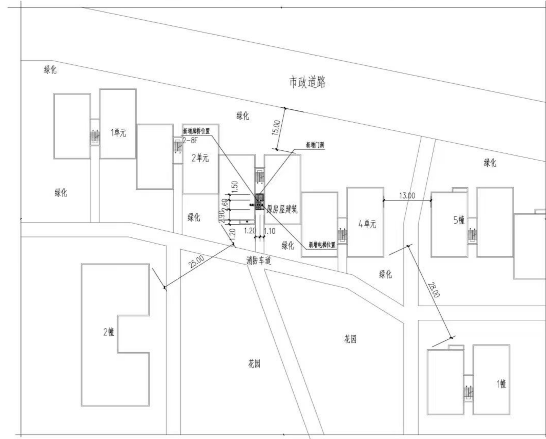
总平面图 1:500
