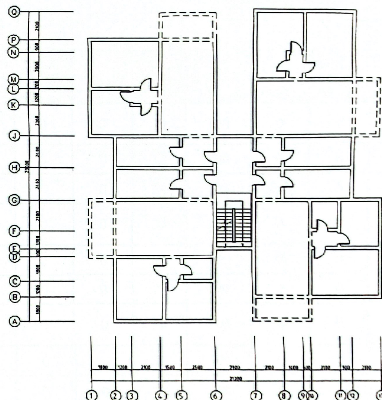
1-8 层平面布置图
