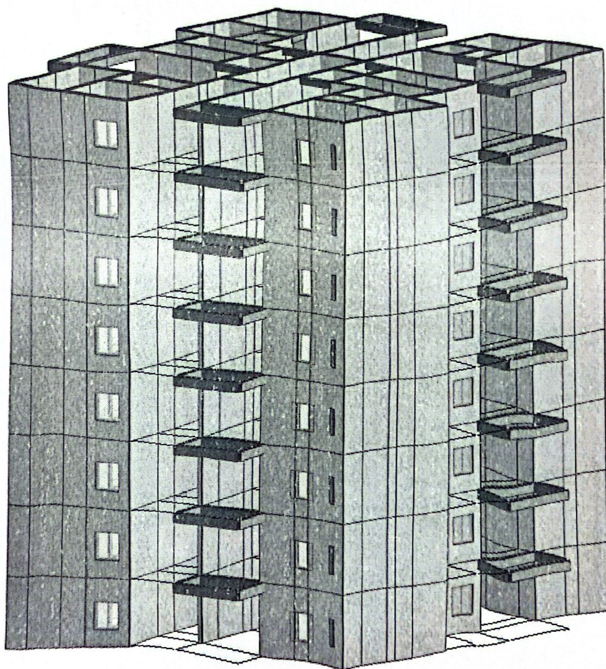
图 4-1 结构验算计算模型
