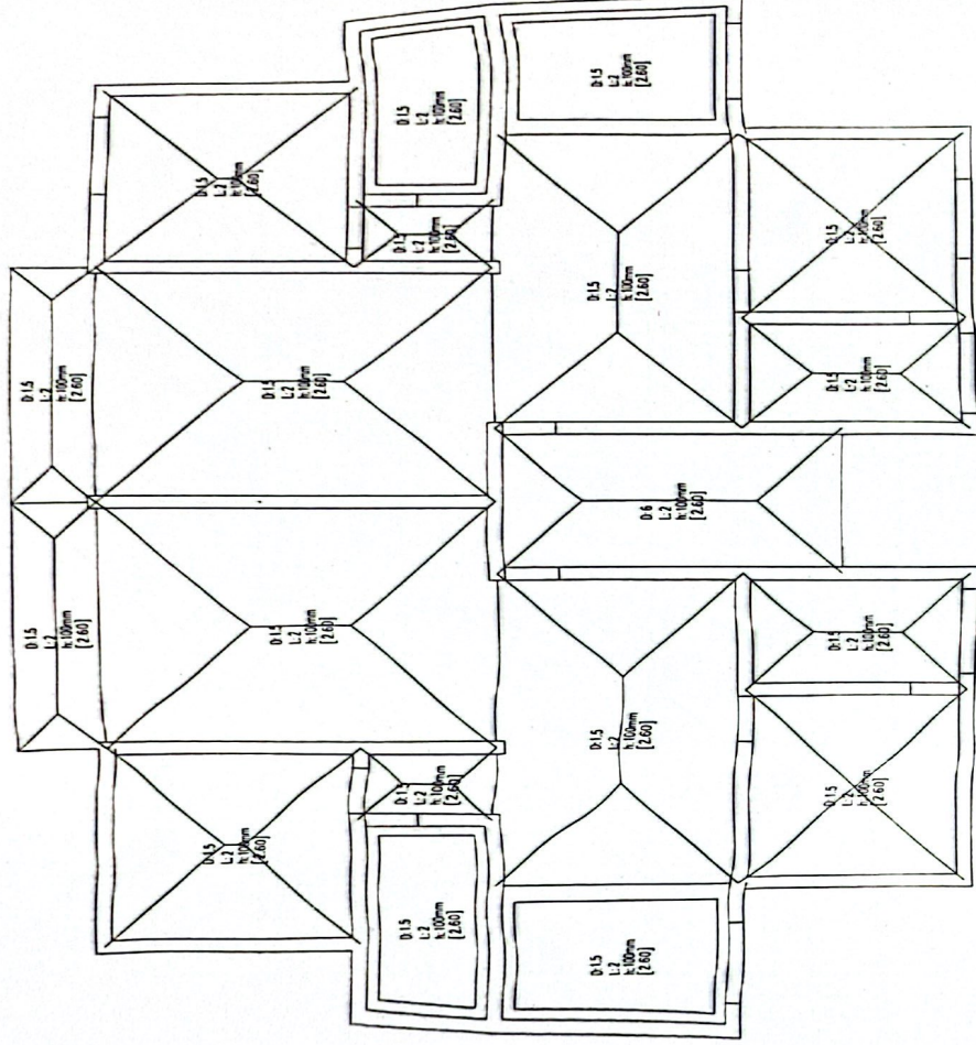
L2 平面荷载简图
