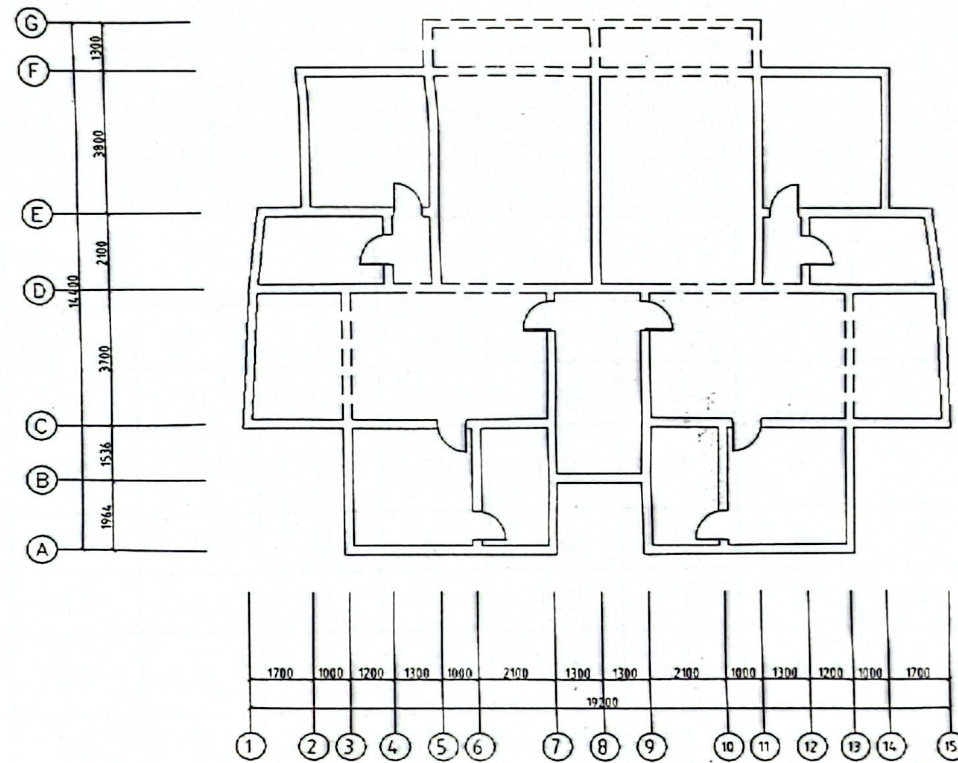
1-7层平面布置图
