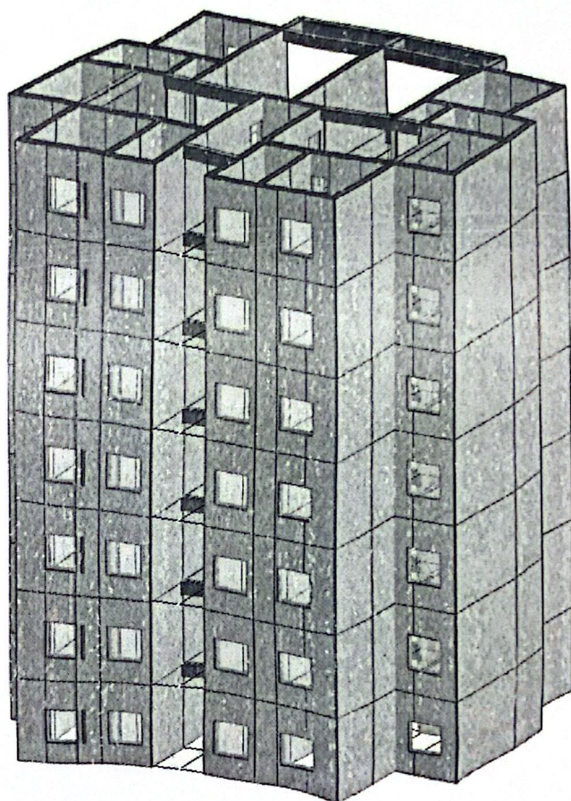
图 4-1 结构验算计算模型
