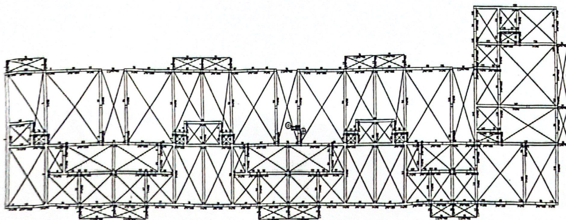
图 4-5 四层主要构件截面尺寸
