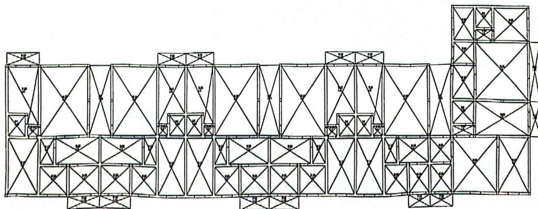
图 4-11 二层荷载简图
