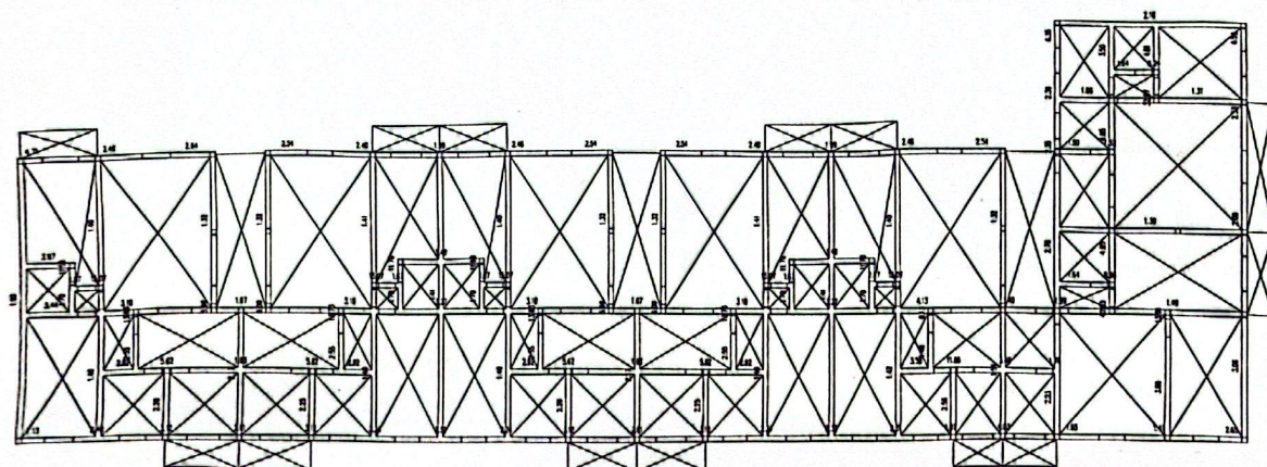
图 5-3 三层受压承载力计算结果
