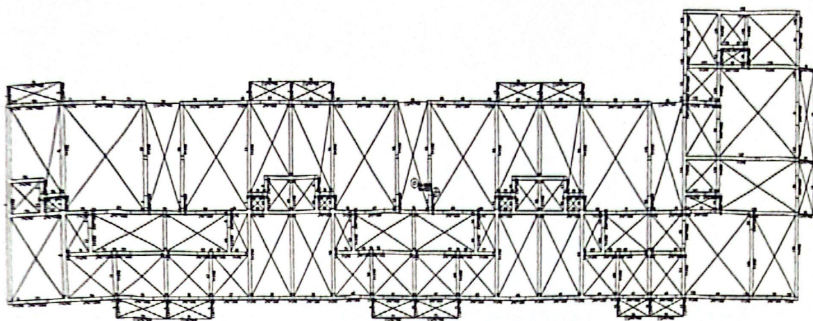
图 4-3 二层主要构件截面尺寸
