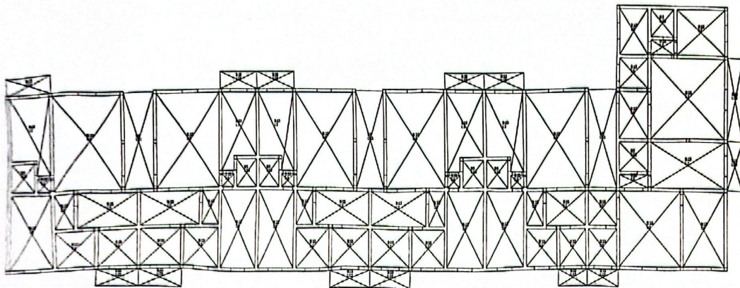
图 4-16 七层荷载简图
