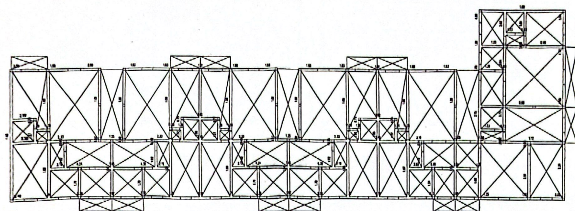
图 5-1 一层受压承载力计算结果
