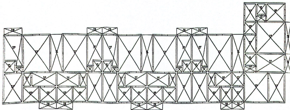
图 4-10 一层荷载简图
