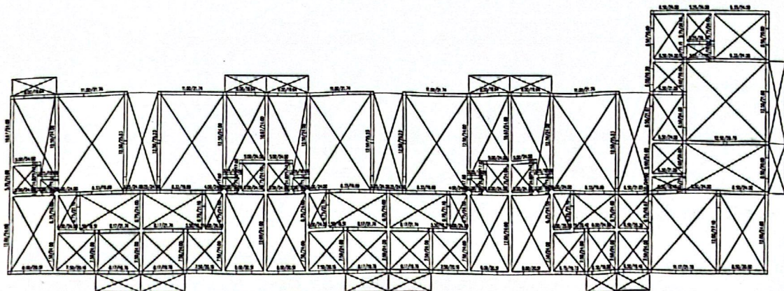
图 5-12 四层高厚比计算结果
