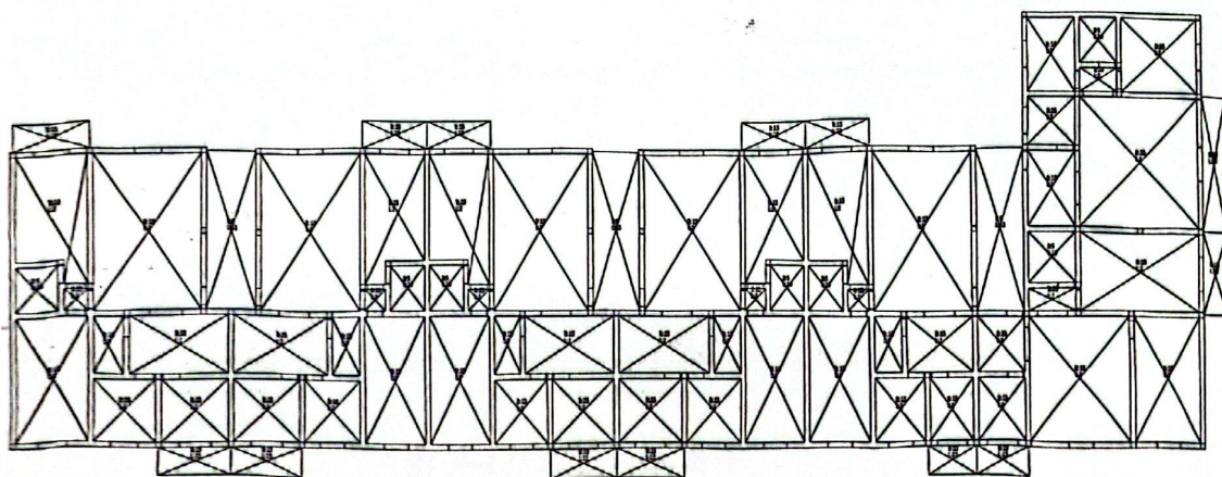
图 4-14 五层荷载简图
