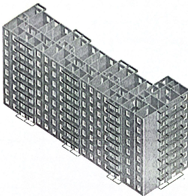
图 4-1 结构验算计算模型
