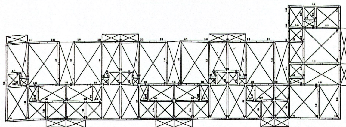
图 5-2 二层受压承载力计算结果
