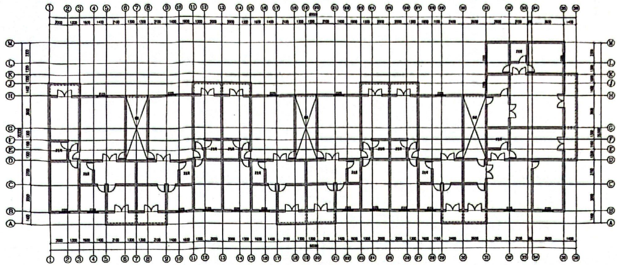
一层~八层平面示意图
