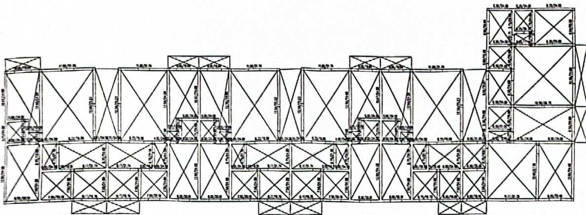
图 5-11 三层高厚比计算结果
