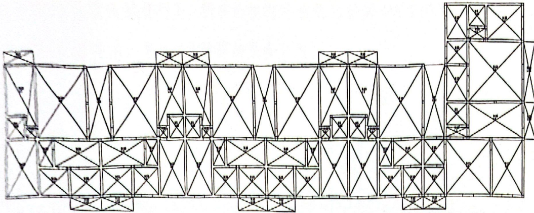
图 4-15 六层荷载简图
