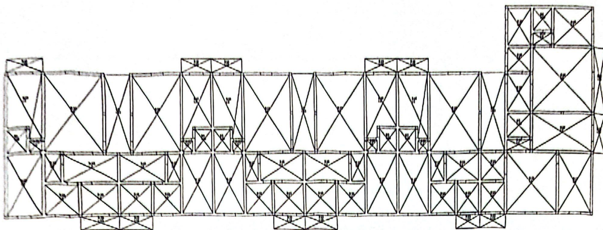
图 4-12 三层荷载简图
