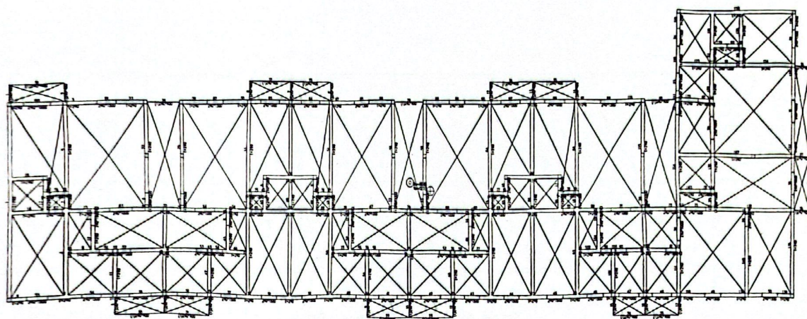
图 4-7 六层主要构件截面尺寸
