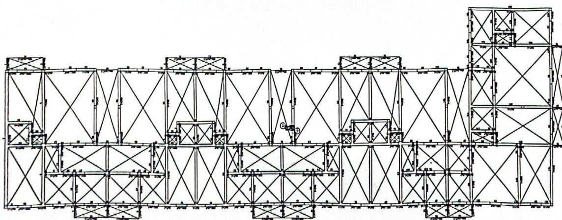
图 4-2 一层主要构件截面尺寸
