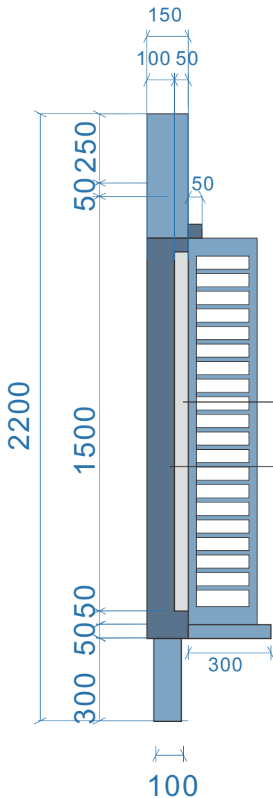
侧面图
