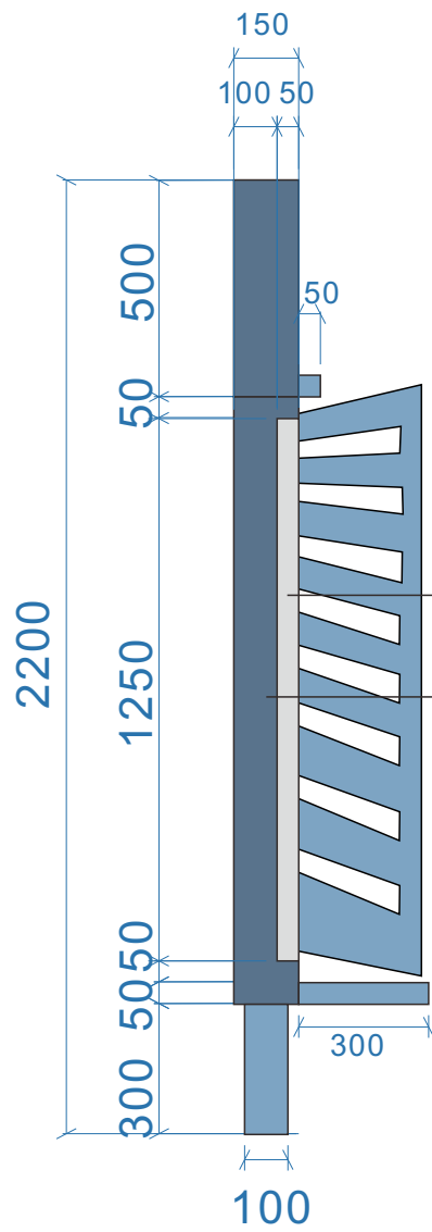
侧面图
