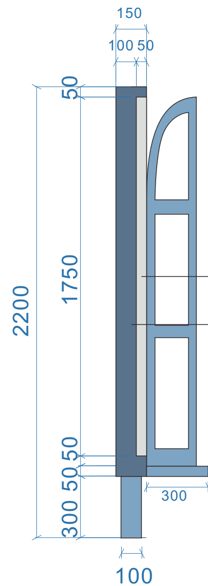
侧面图
