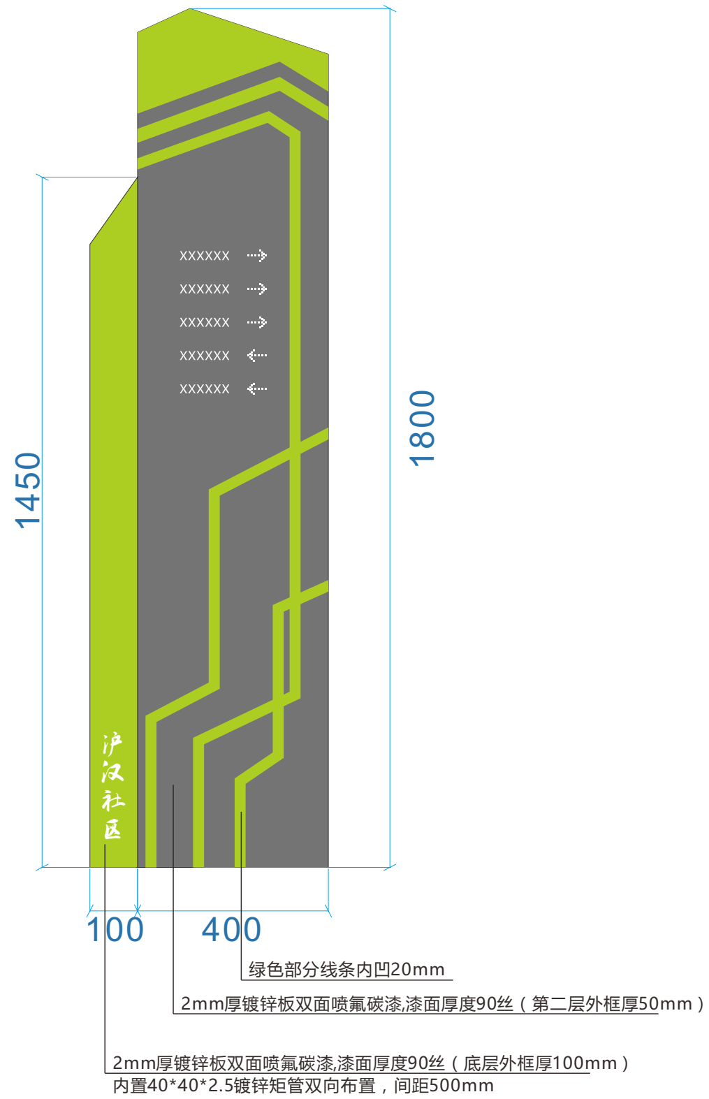
立面图
