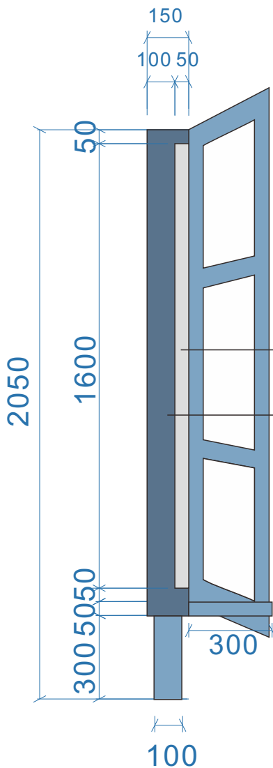
侧面图
