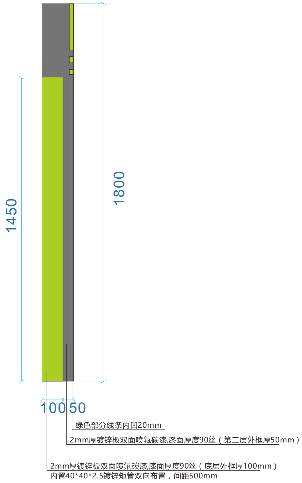
侧面图
