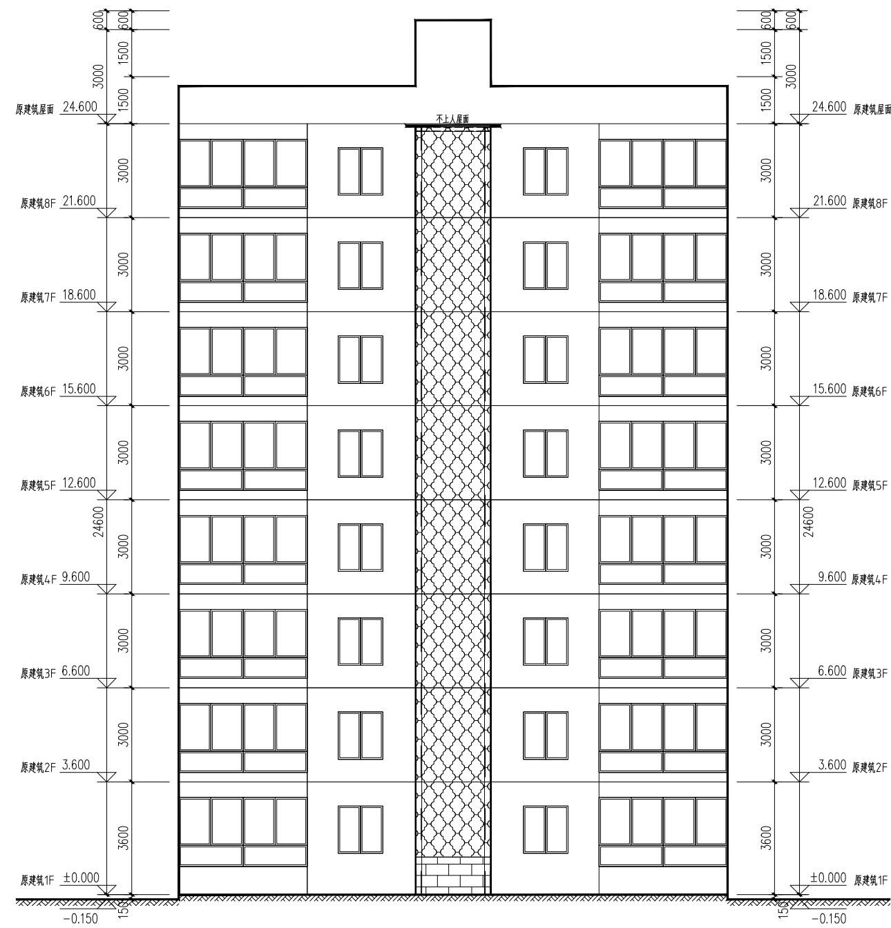
增设电梯立面示意图 1:100
