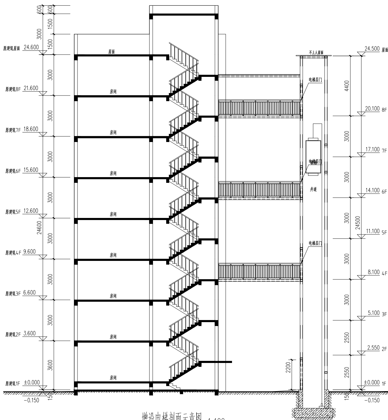
增设电梯剖面示意图 1:100
