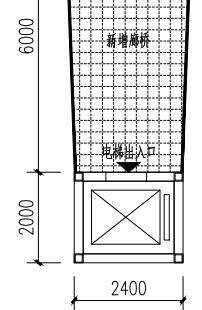
增设电梯标准层示意图 1:100
