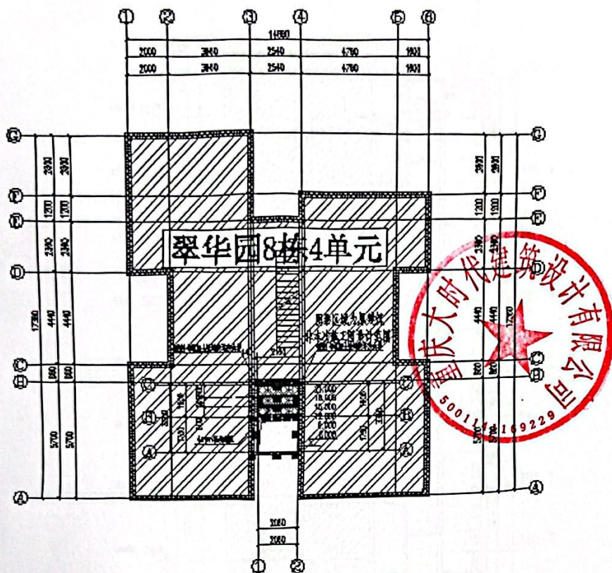
图 2-1 新增电梯标准层结构平面图
