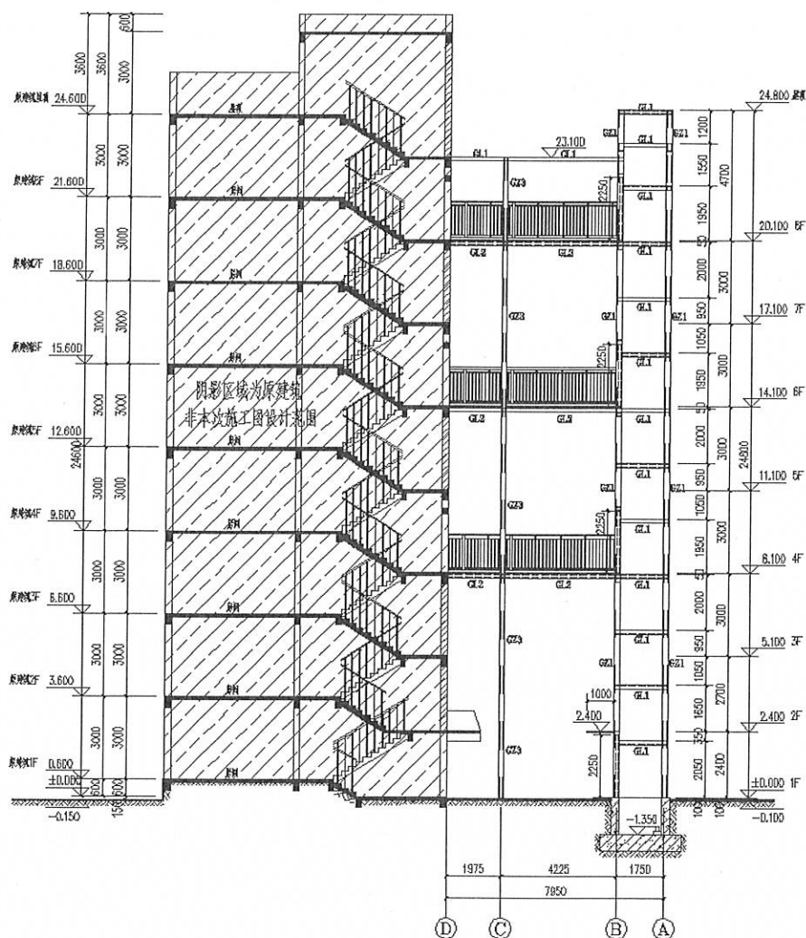
图 2-2 新增电梯标准层结构立面布置
